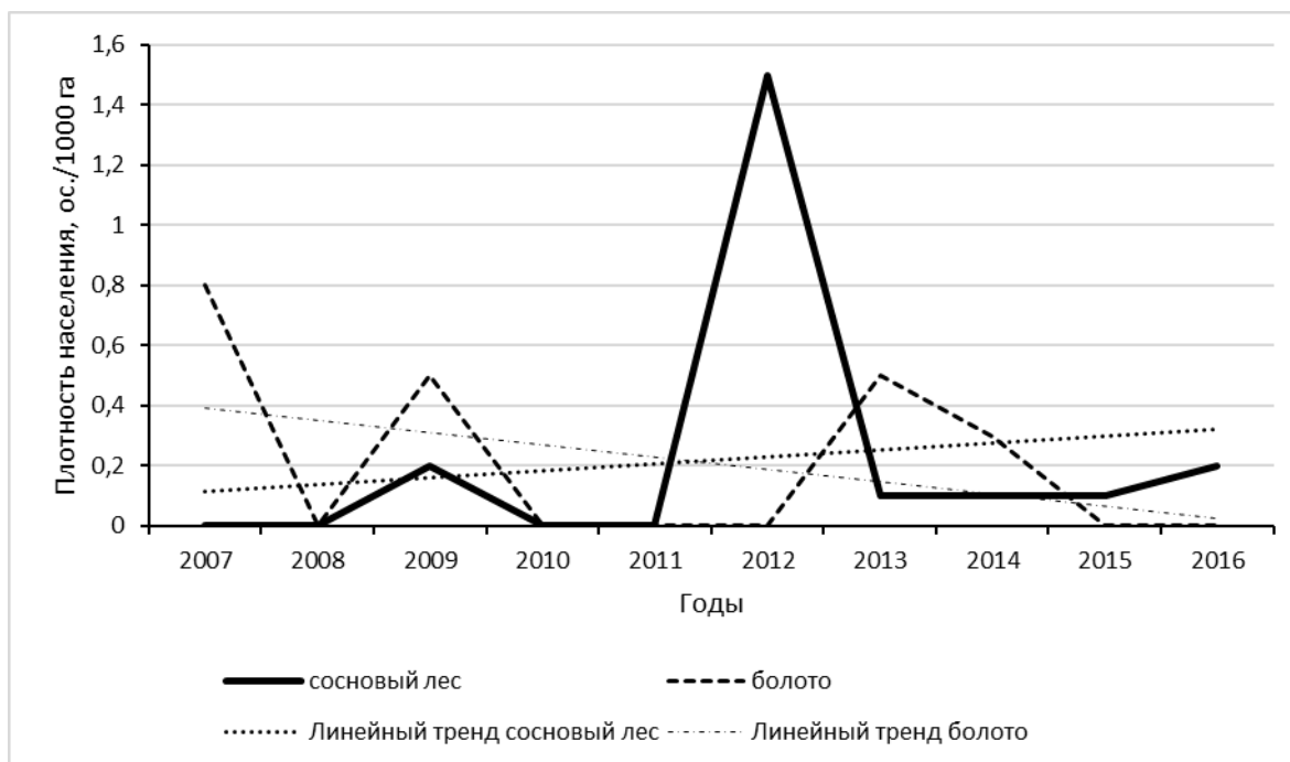
Рис. 2. Динамика численности популяции северного оленя в сосновых и болотных биотопах заповедника «Юганский» по результатам ЗМУ (2007–2016 гг.)
